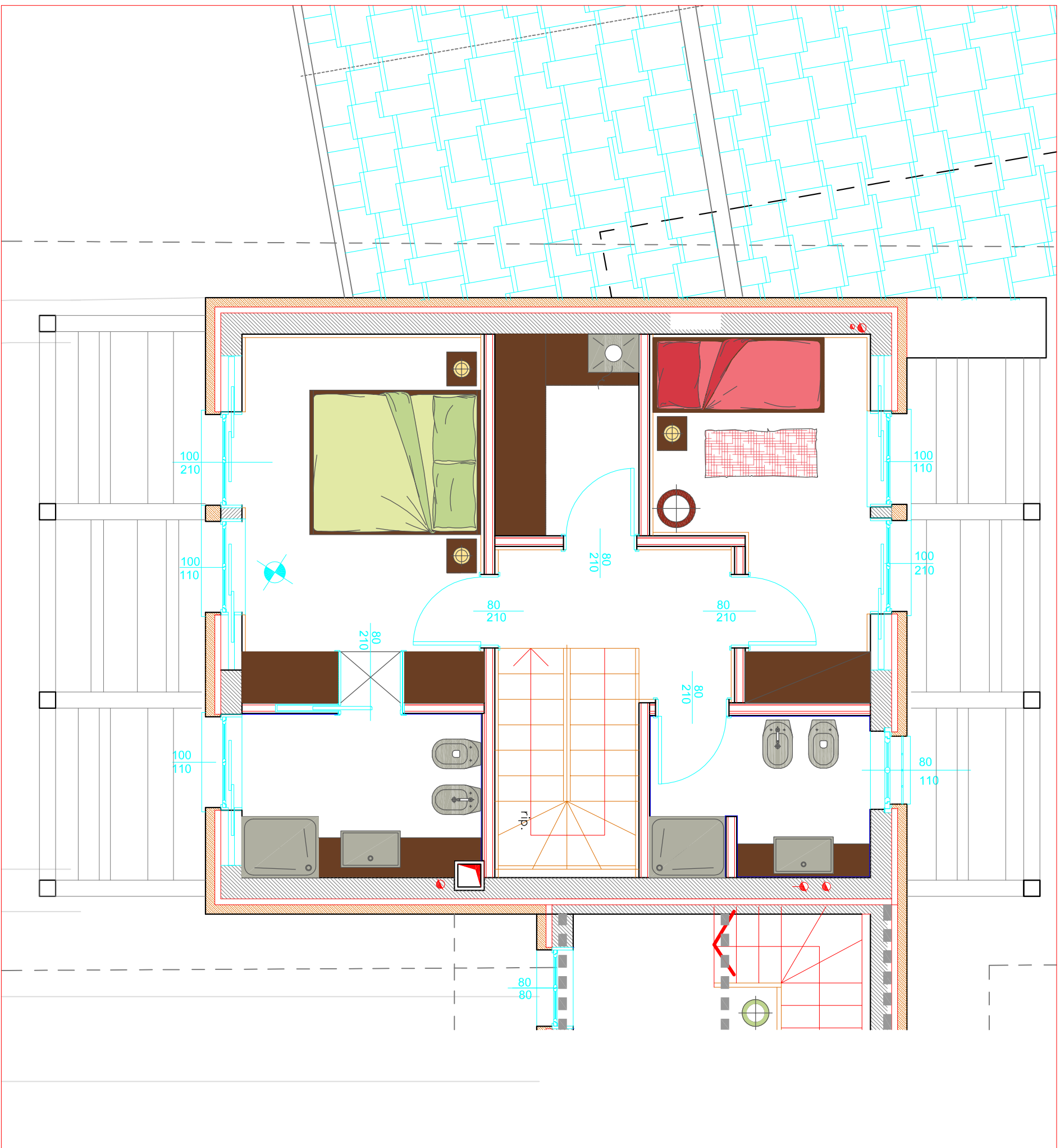
PIANTA PIANO PRIMO SCALA 1:50
